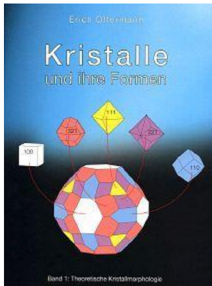
Die Kristallformen
