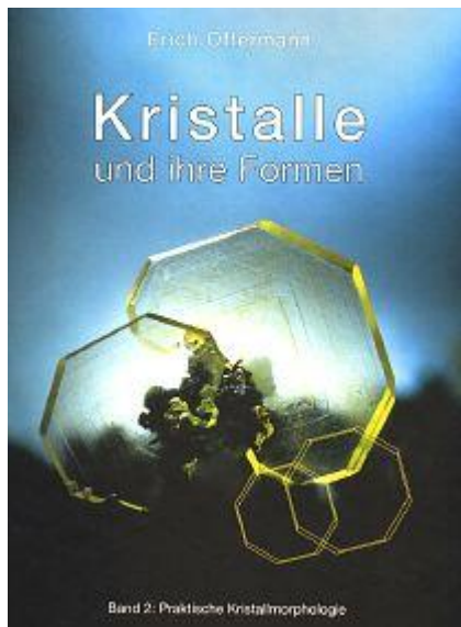
Wunderbare Einzelkristalle
